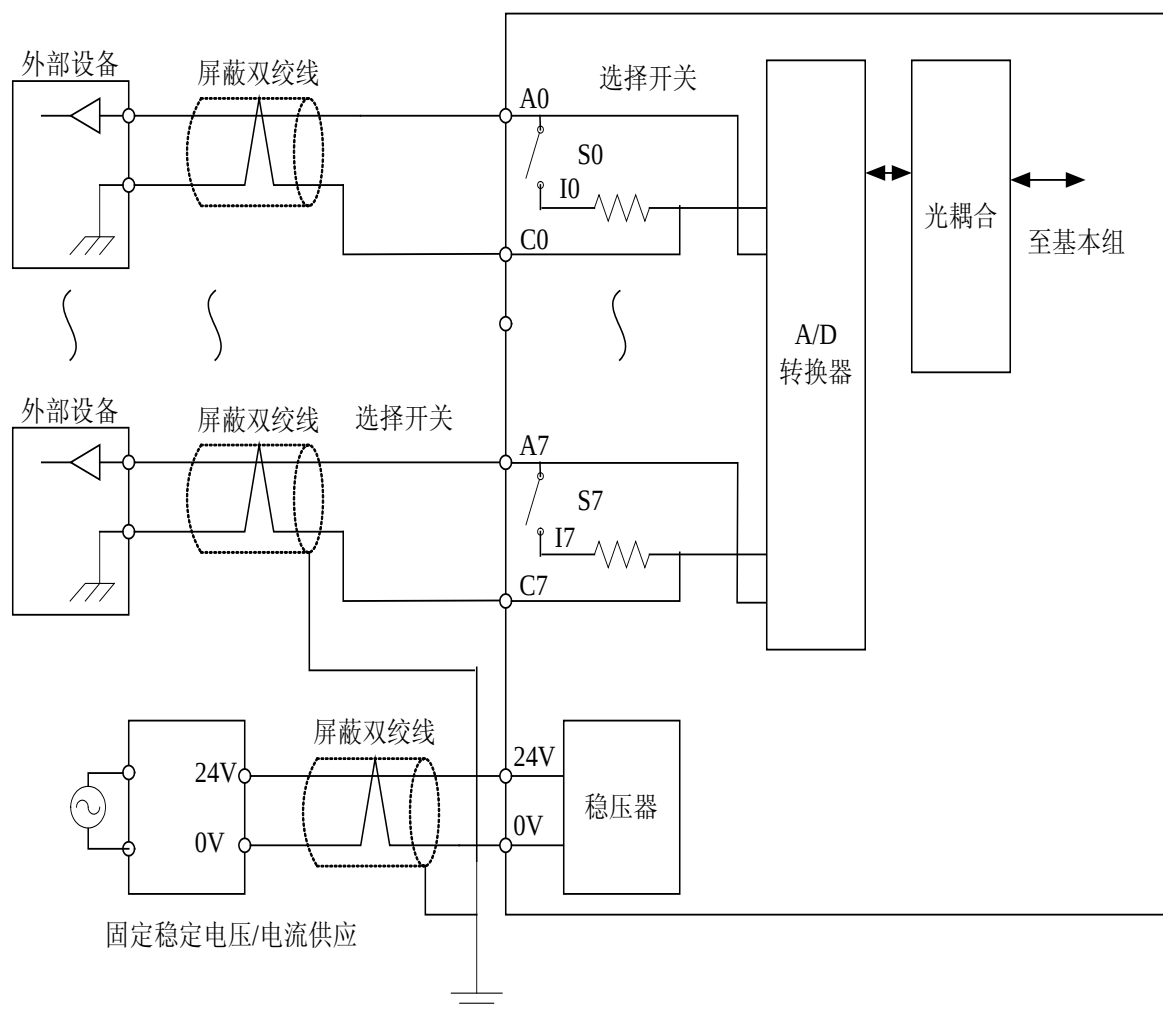
回路图
