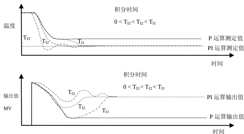
示例 2: 冷却（正动作）时的 PI 运算
