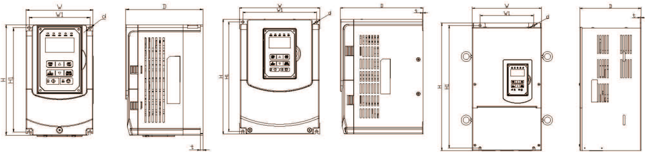
外型图 A
