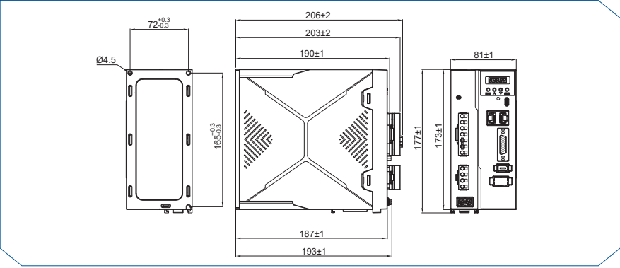
JSDL3-15B/25B/35B (-E) 产品尺寸
