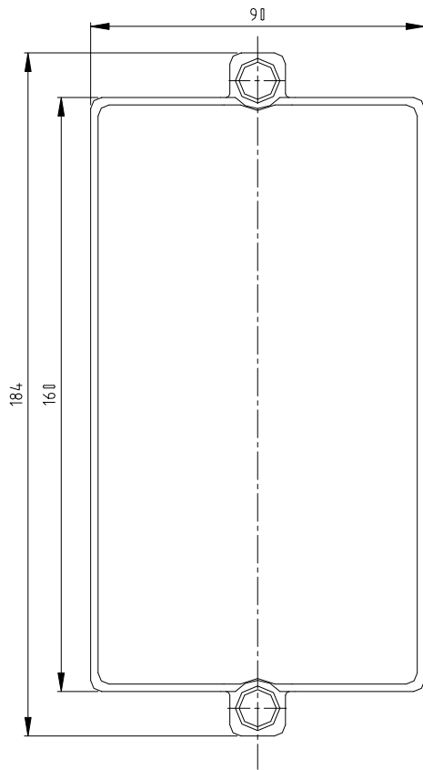
HUF-11/16 外型圖
