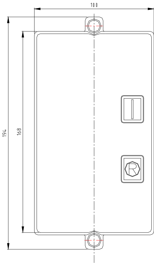
HUPB-18/23 外型圖
