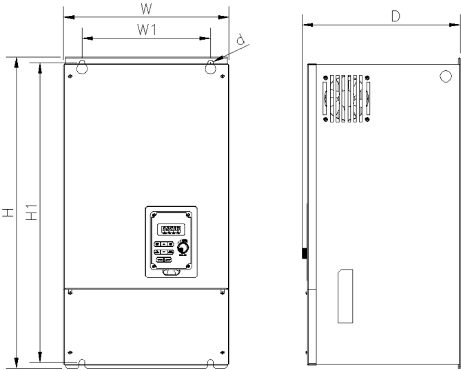
(d) 380V :40-75HP (IP20)
