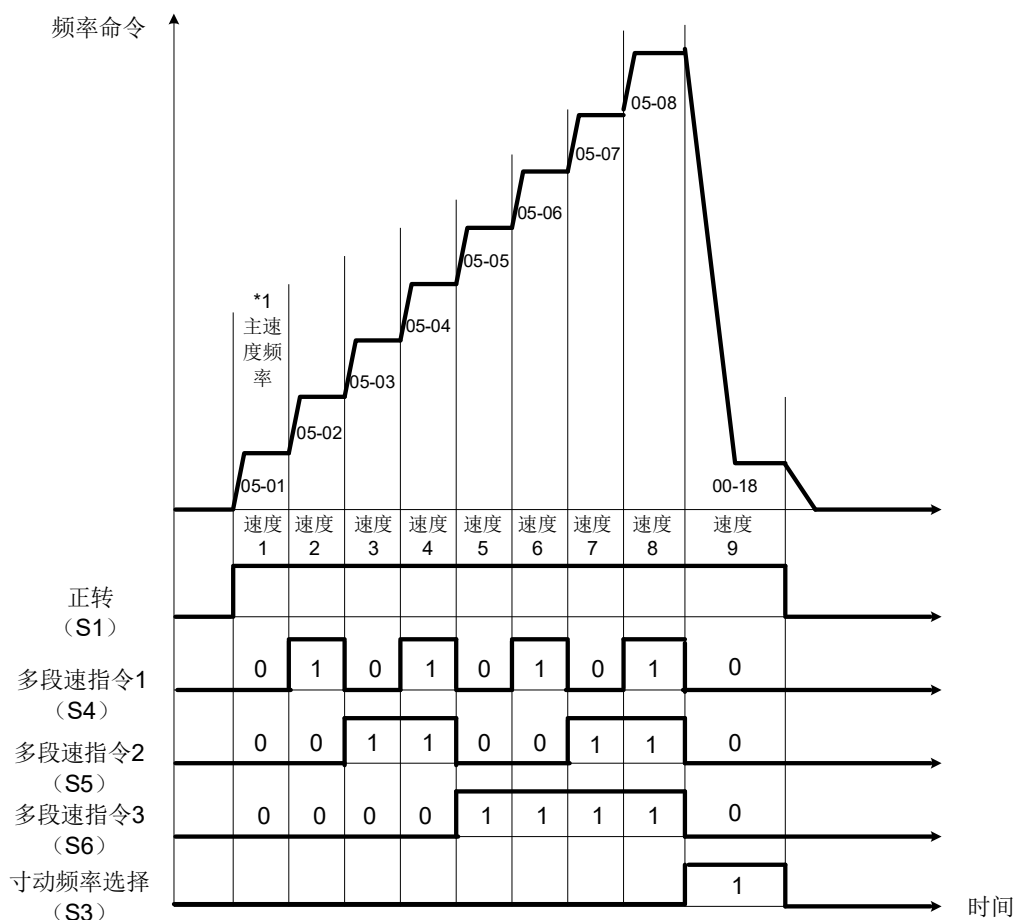
9段速时序图
