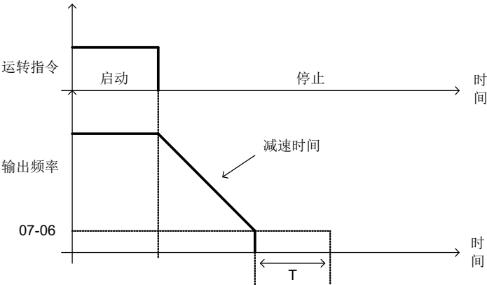
T: 停止时直流刹车时间 (07-08)
