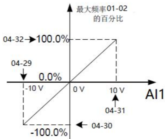
频率给定有负值的设置
