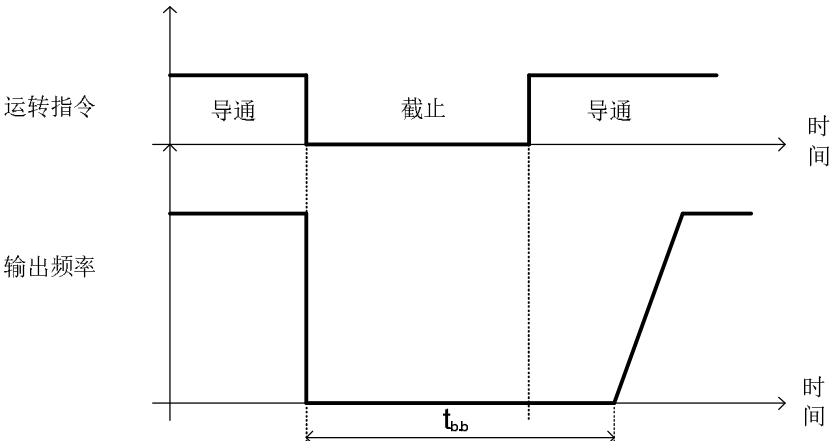
最小基极遮断时间(07-18)
