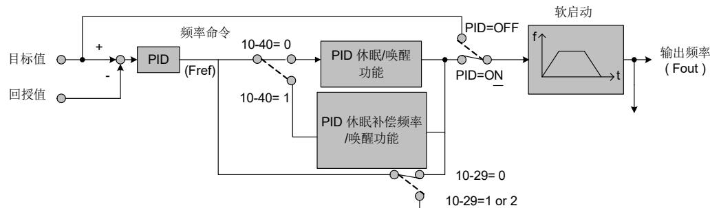
(a) PID 控制方块图
