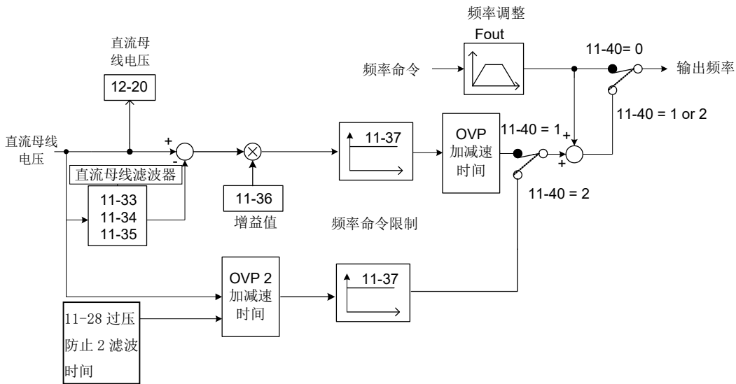
图 4.3.88 OVP操作
