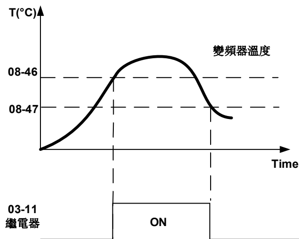
变频器温度到达及复归侦测
