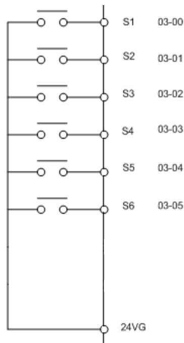
图 4.3.16 多功能数字输入与相关参数
