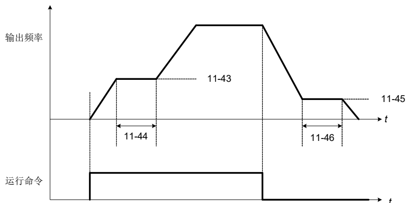
图 4.3.91 保持功能
