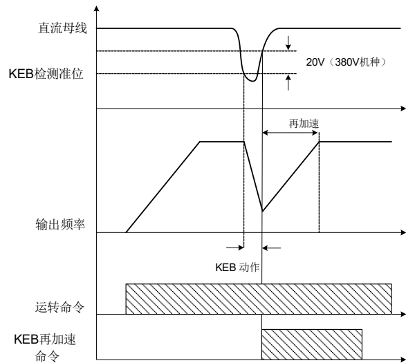
· 图 4.3.92 KEB 操作
