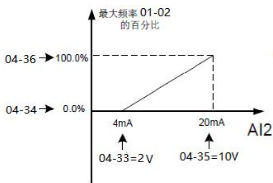
频率给定没有负值时的设置
