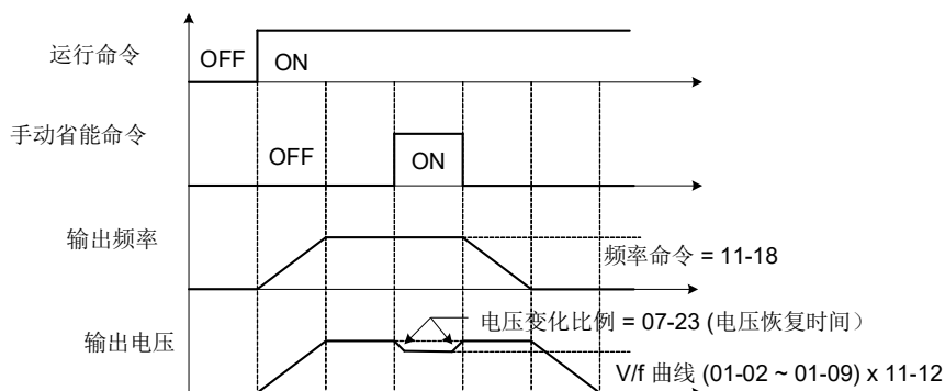
图 4.3.85 手动节省能源操作
