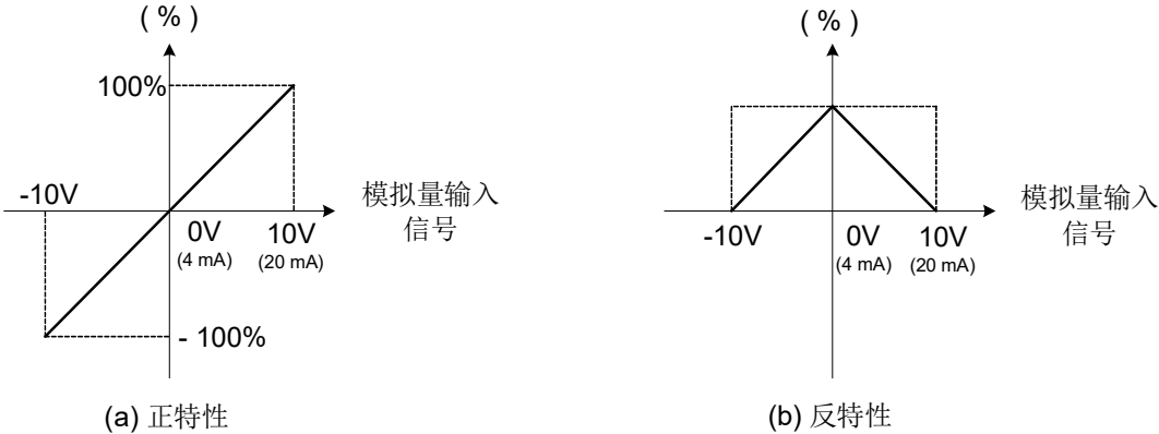
图 4.3.10 主要频率参考之正/反特性
