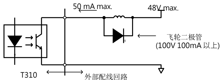
图 3.5 光耦合输出接点接电感性负载
