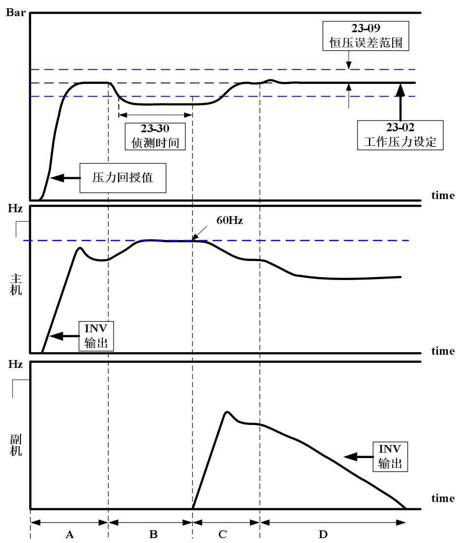
图 4.3.109 双泵浦启动功能流程
