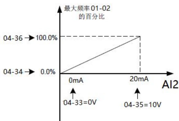
频率给定没有负值时的设置 (默认设置)
