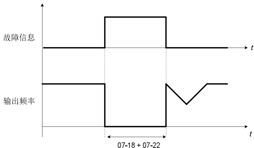
图 4.3.52 自动复归再启动操作
