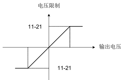
图 4.3.86 调机操作电压限制值
