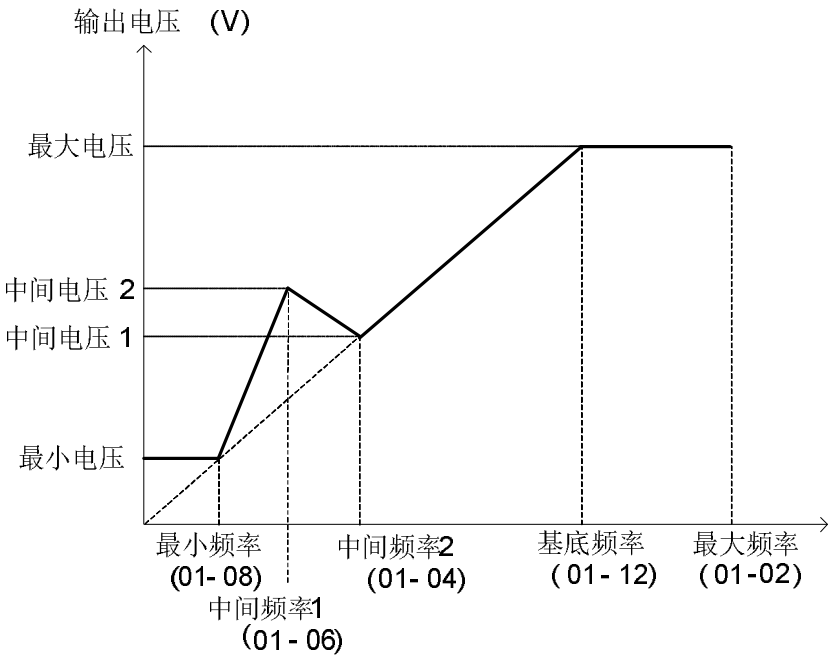
图 4.3.13 转矩提升
